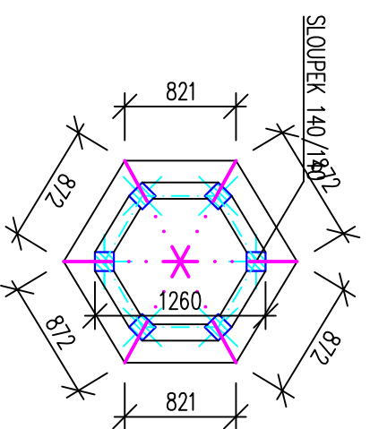
PŮDORYS KROVU
