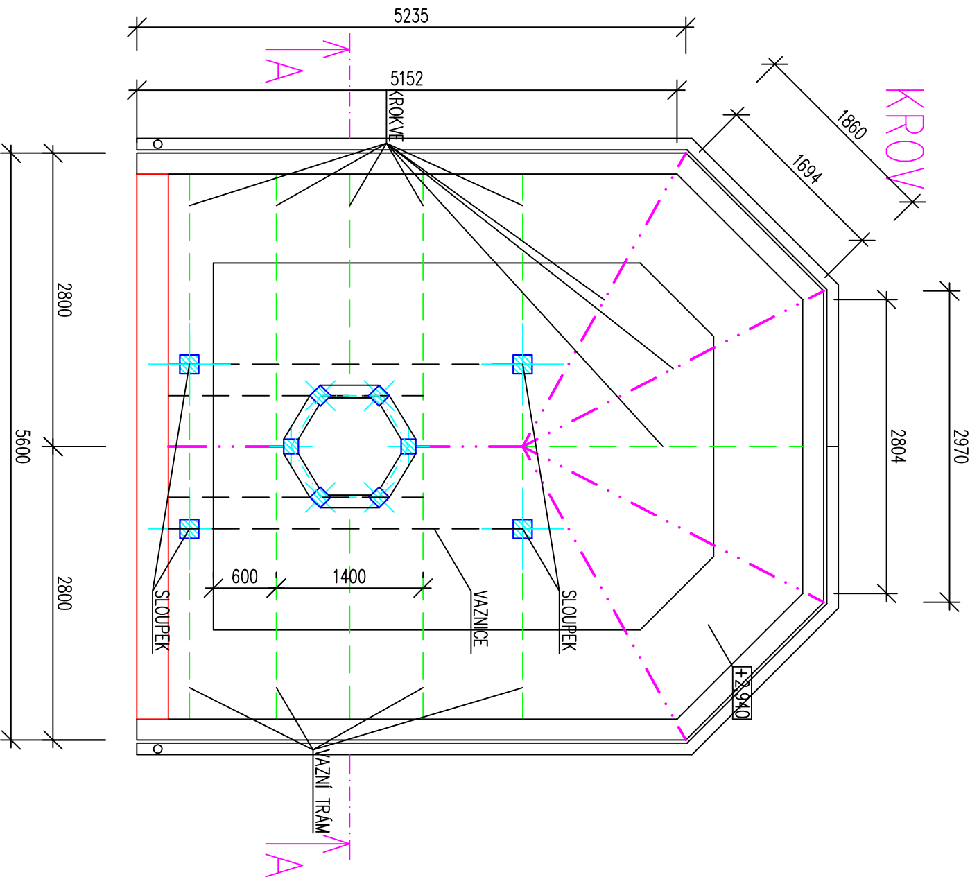
PŮDORYS KROVU
